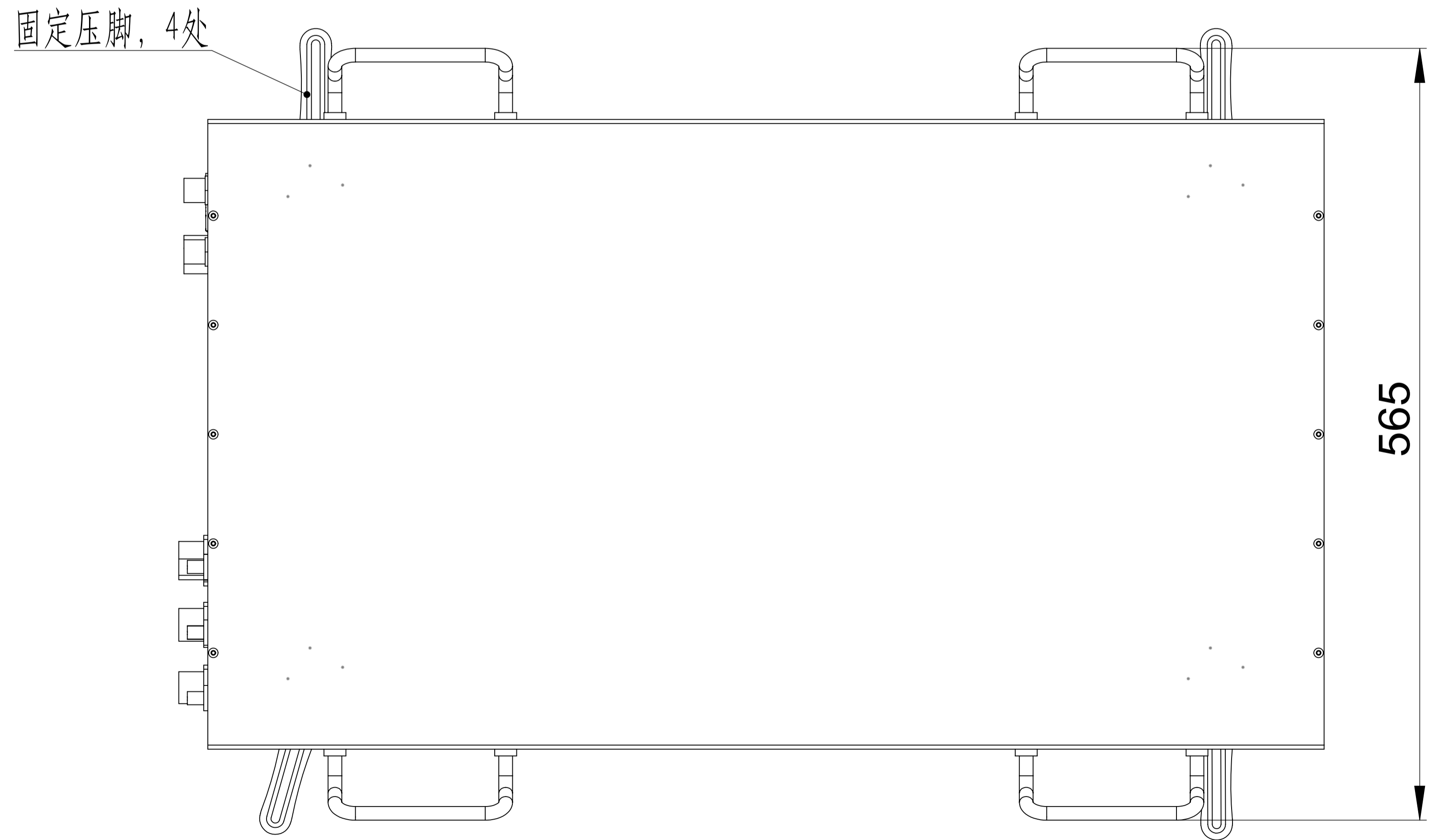
俯视图
