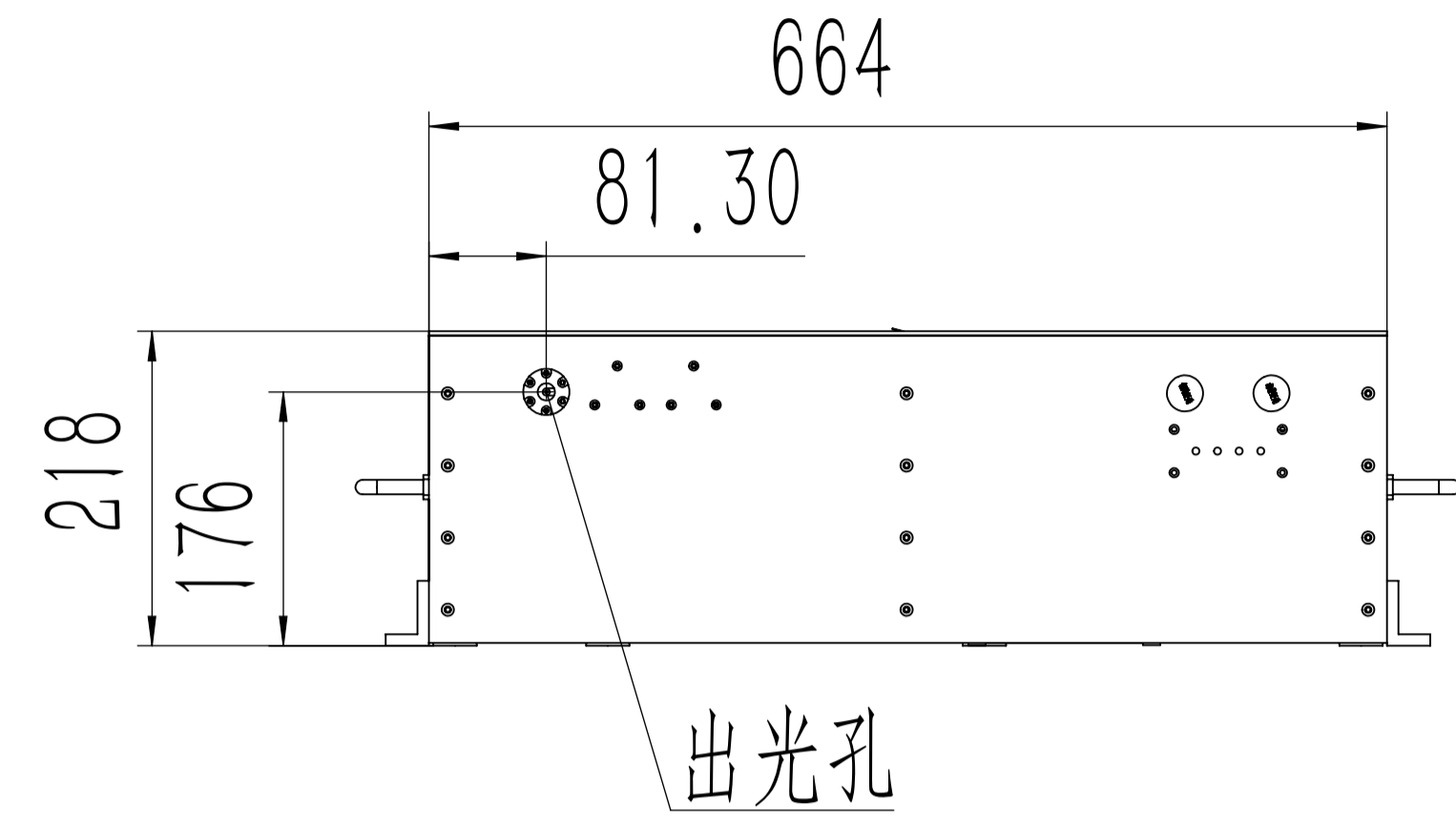
前视图
