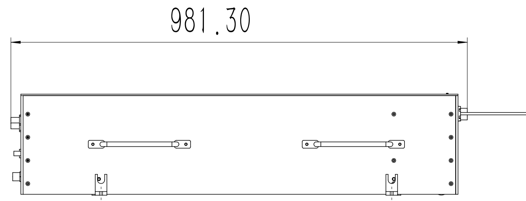
侧视图
