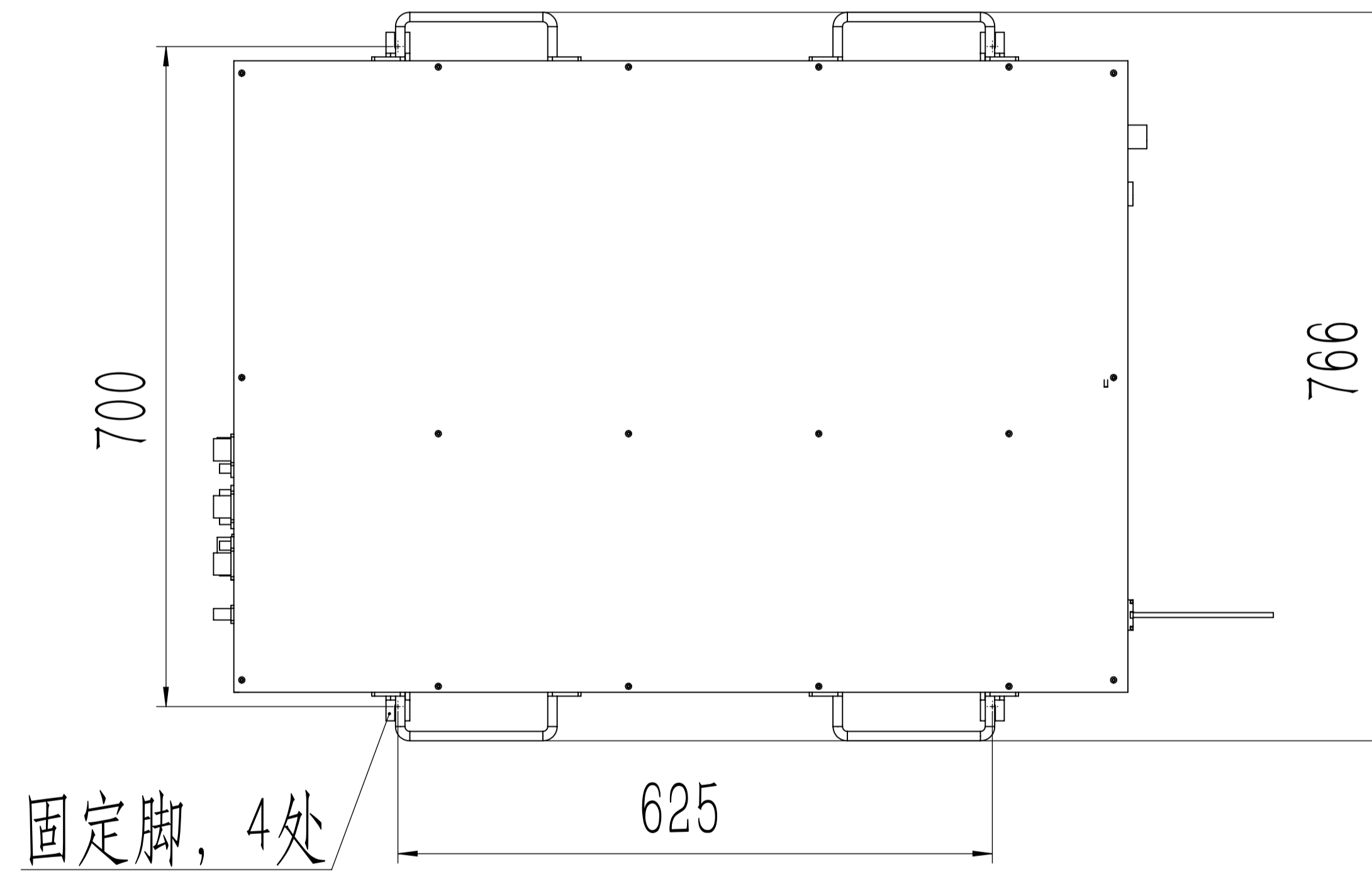
上视图
